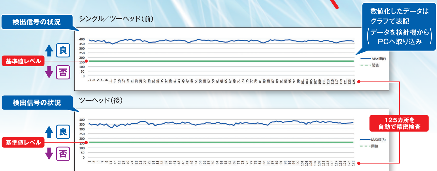
ハシマツーヘッド検針機の検出グラフ
